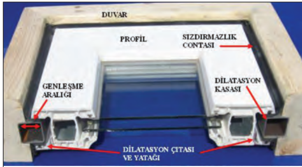
Resim 4. Vidasız Montaj Metodu Bileşenleri ve Detayı[3]
