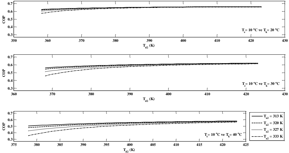
Şekil 4. ADS Sistemin COP Değerinin Farklı Kondanser ve 10 °C Evaporatör Sıcaklığı İçin Desorpsiyon ve Adsorpsiyon Sıcaklıkları İle Değişimi.
