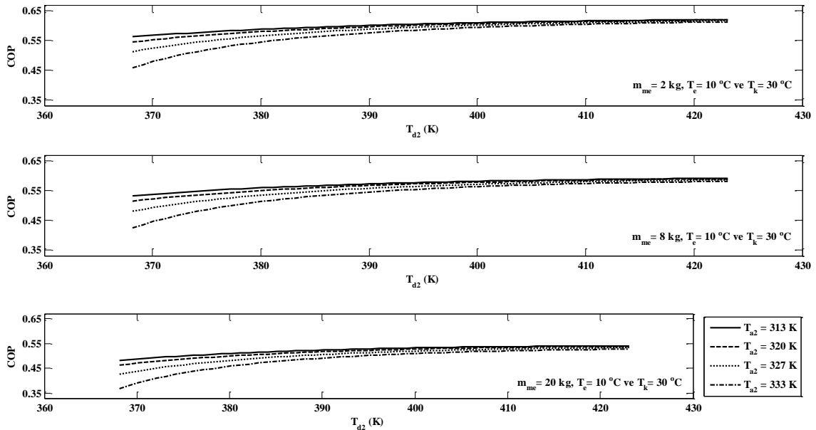
Şekil 6. ADS Sistemin COP Değerinin Farklı Metal Kütle Değerleri İçin Desorpsiyon ve Adsorpsiyon Sıcaklıkları İle Değişimi.
