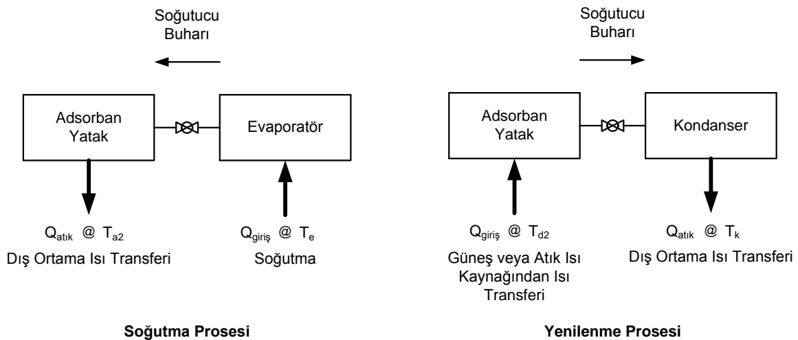
Şekil 1. Basit ADS Sisteminin Şematik Gösterimi.
