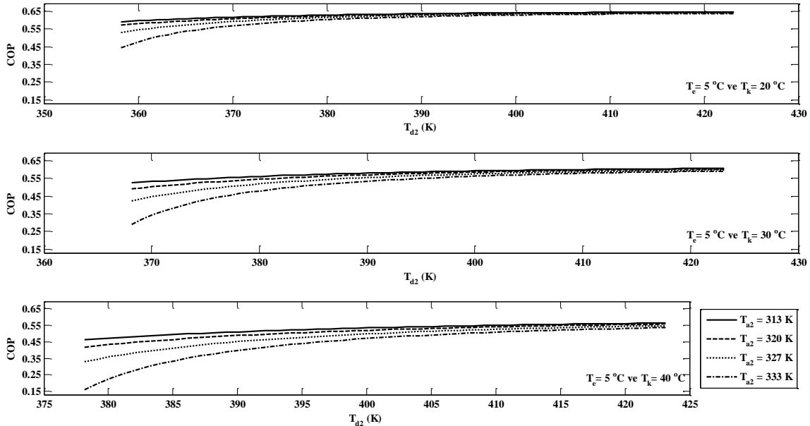
Şekil 3. ADS Sistemin COP Değerinin Farklı Kondanser ve 5 °C Evaporatör Sıcaklığı İçin Desorpsiyon ve Adsorpsiyon Sıcaklıkları İle Değişimi.
