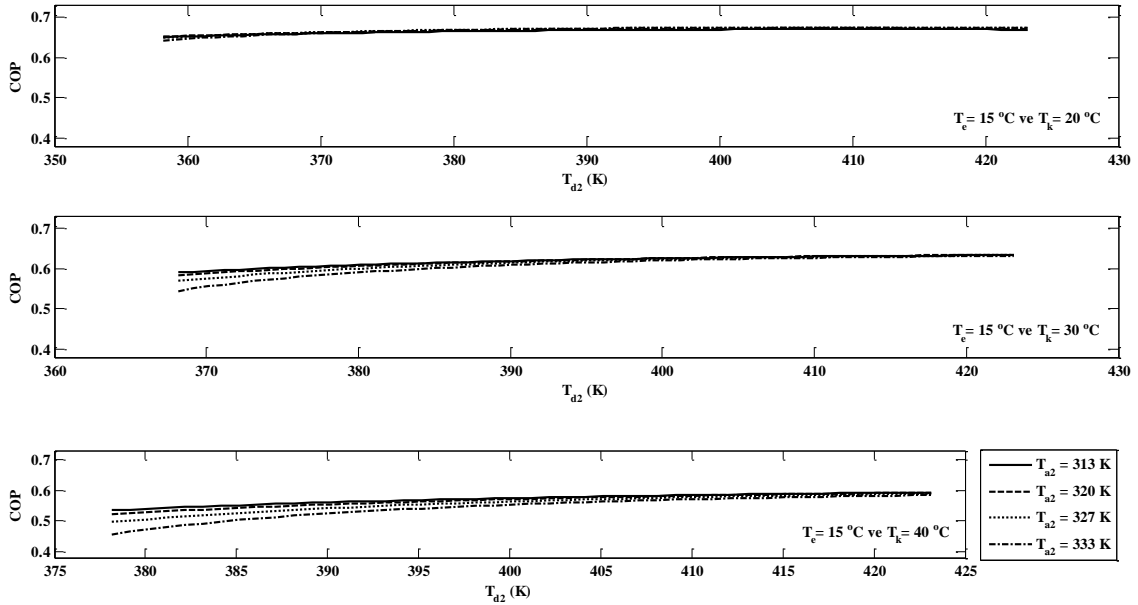
Şekil 5. ADS Sistemin COP Değerinin Farklı Kondanser ve 15 °C Evaporatör Sıcaklığı İçin Desorpsiyon ve Adsorpsiyon Sıcaklıkları İle Değişimi.
