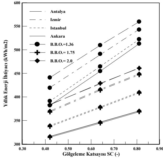
Şekil 2. Gölgeleme Katsayısının Yıllık Enerji İhtiyacına Olan Etkisi.
