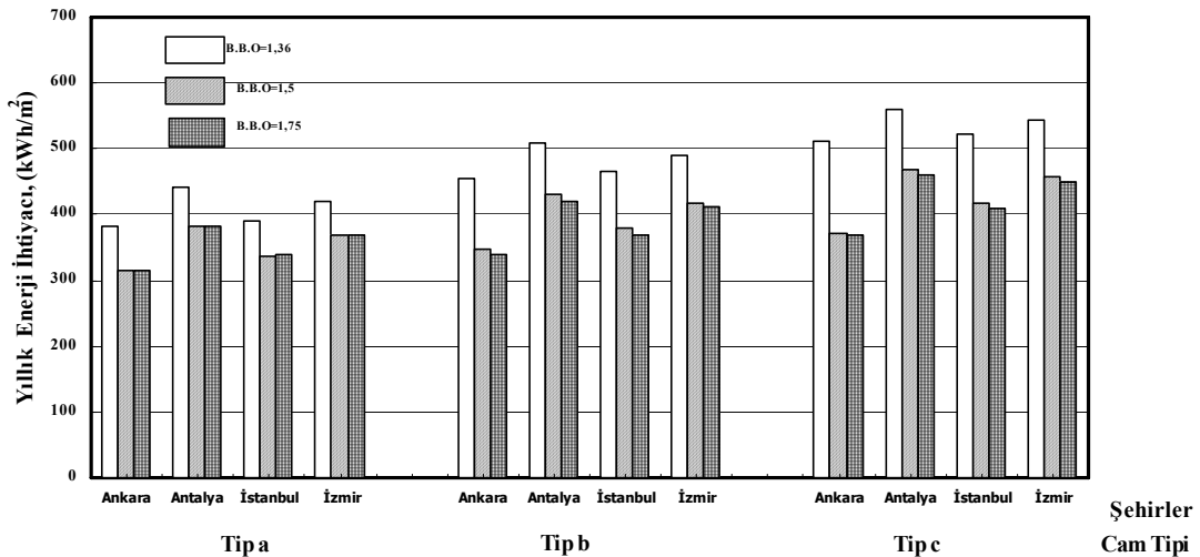
Şekil 1. Farklı Cam Tiplerinin Enerji İhtiyacı Üzerindeki Etkisi.
