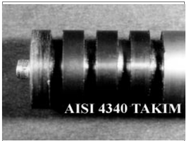
Şekil 2. FSW Yöntemi Uygulanarak Yapılan Deneylerde Kullanılan Takımın Görünümü (19).
