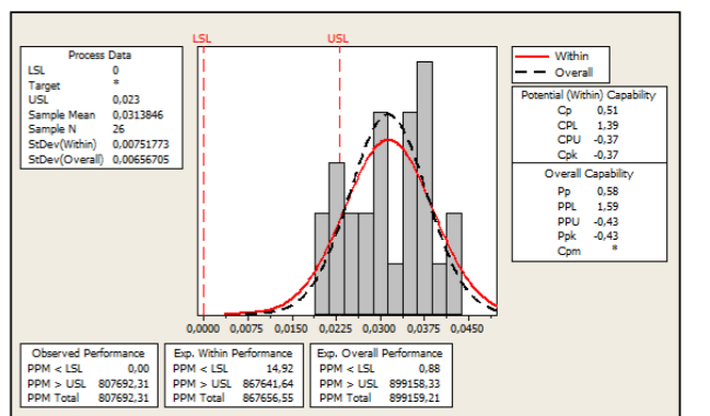
Şekil 8. Süreç Yeterlilik Analiz Grafiği
