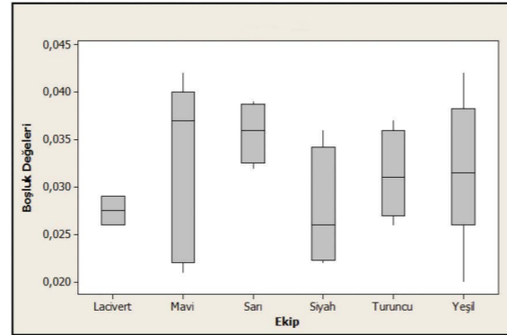
Şekil 10. Teknisyene Göre Boşluk Değeri Kutu Grafiği
