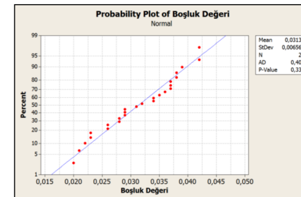
Şekil 7. Boşluk Değerleri İçin Normalite Testi Grafiği
