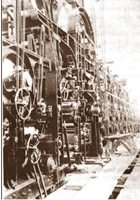
Mehmet Ali Kaçitçi objektifinden fabrikadaki 1 numaralı kâğıt makinasının kurutma kısmı
