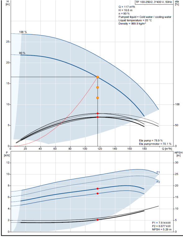
6" ARMATÜR KULLANILMASI HALİNDE POMPA PERFORMANSI
