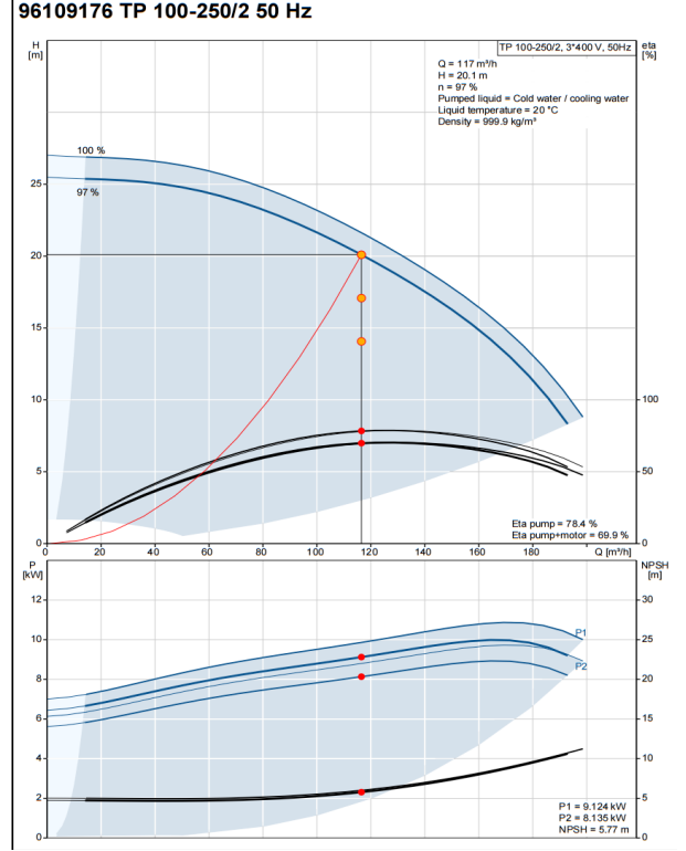
4" ARMATÜR KULLANILMASI HALİNDE POMPA PERFORMANSI
