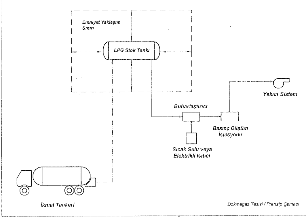
Şekil 1. Dökme LPG Tesisi Prensip Şeması.
