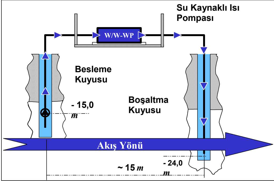
Şekil 8. Sudan suya ısı pompası şeması
