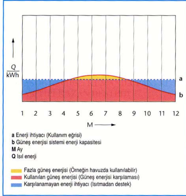
Şekil 10. Kullanma suyu ısıtması için gereken enerjinin güneşten karşılanma oranı
