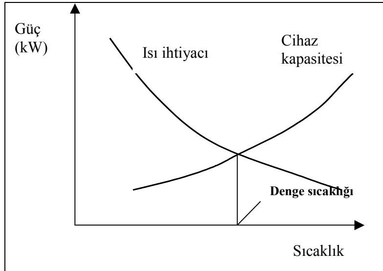
Şekil 7. Denge sıcaklığının şematik tanımı
