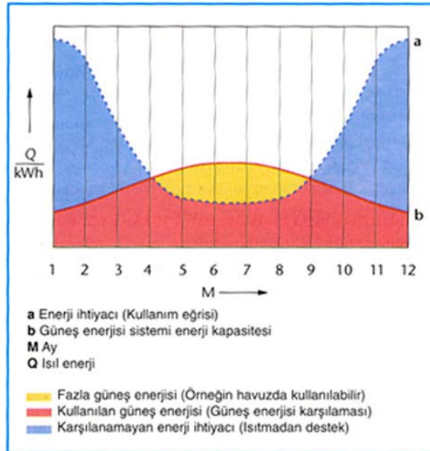
Şekil 11. Isıtmaya destek için güneş enerjisinden yararlanma oranı
