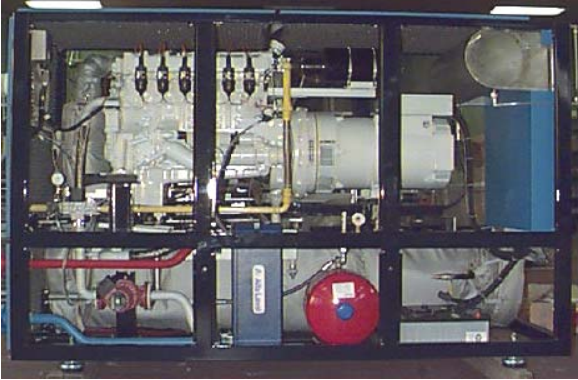
Şekil 16. örnek bir paket kojenerasyon ünitesi iç görüntüsü.
