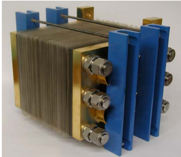
Şekil 14. Prototip yakıt hücresi demeti
