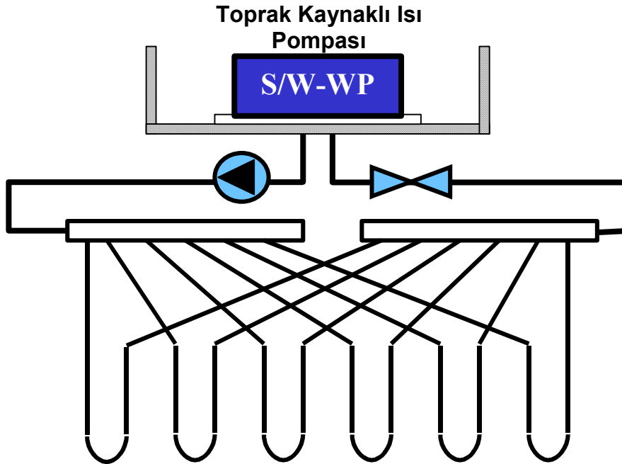
Şekil 9. Toprakta suya ısı pompası şematik gösterimi
