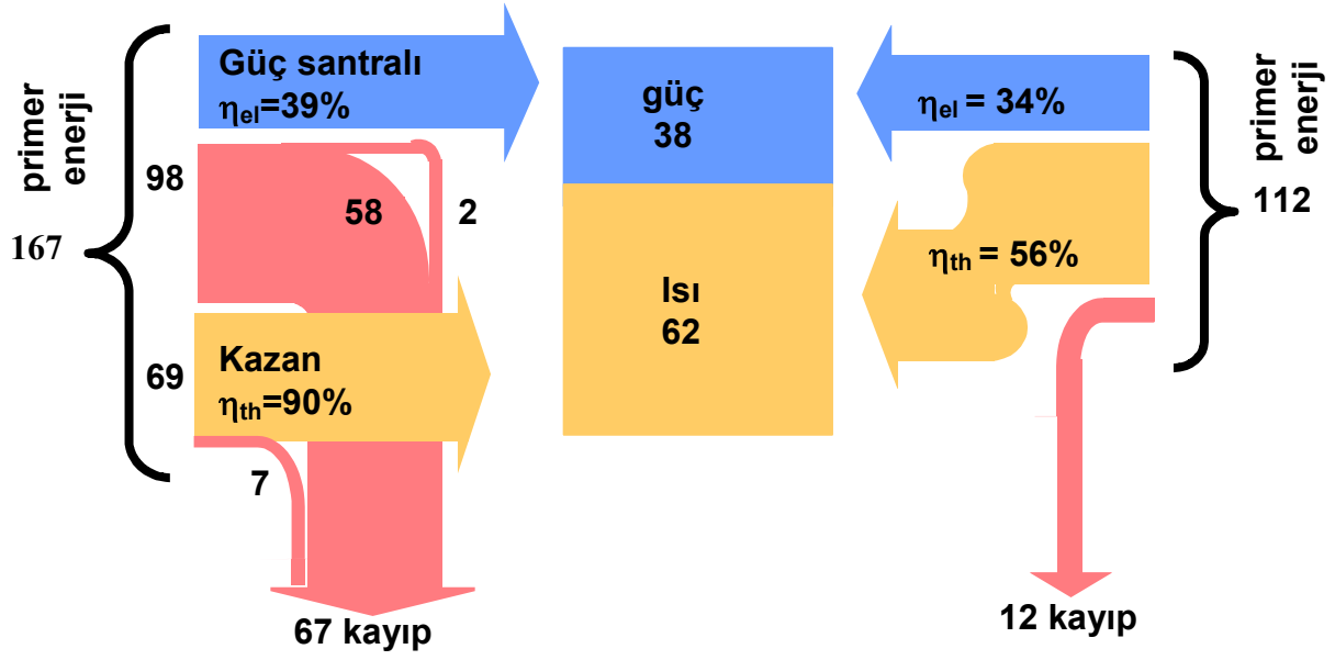
Şekil 15. Kojenerasyon sistemi ve konvansiyonel sistem için enerji akış diyagramı
