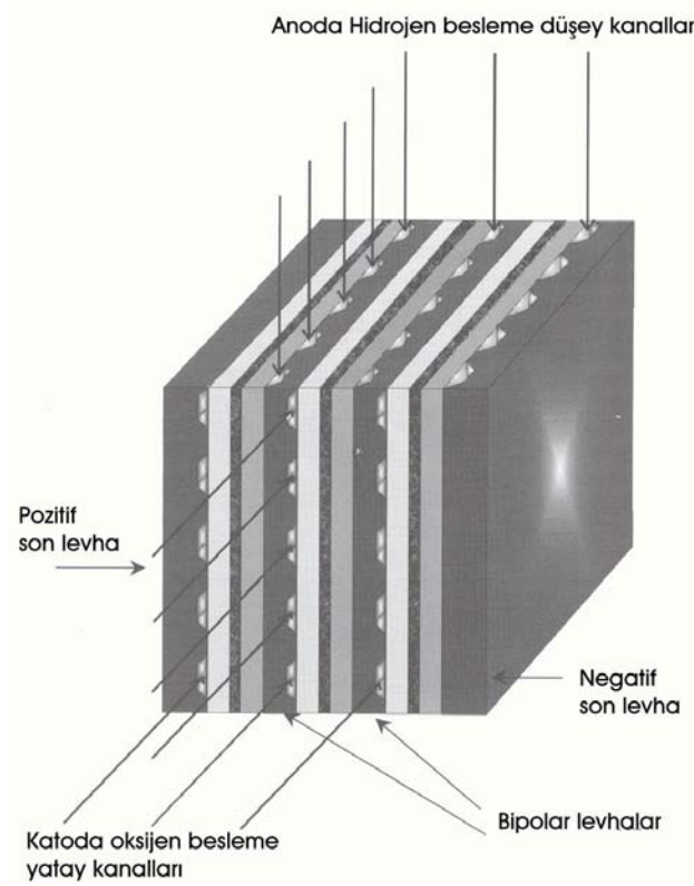
Şekil 13. Üç hücrenin seri bağlantısının şematik gösterilimi
