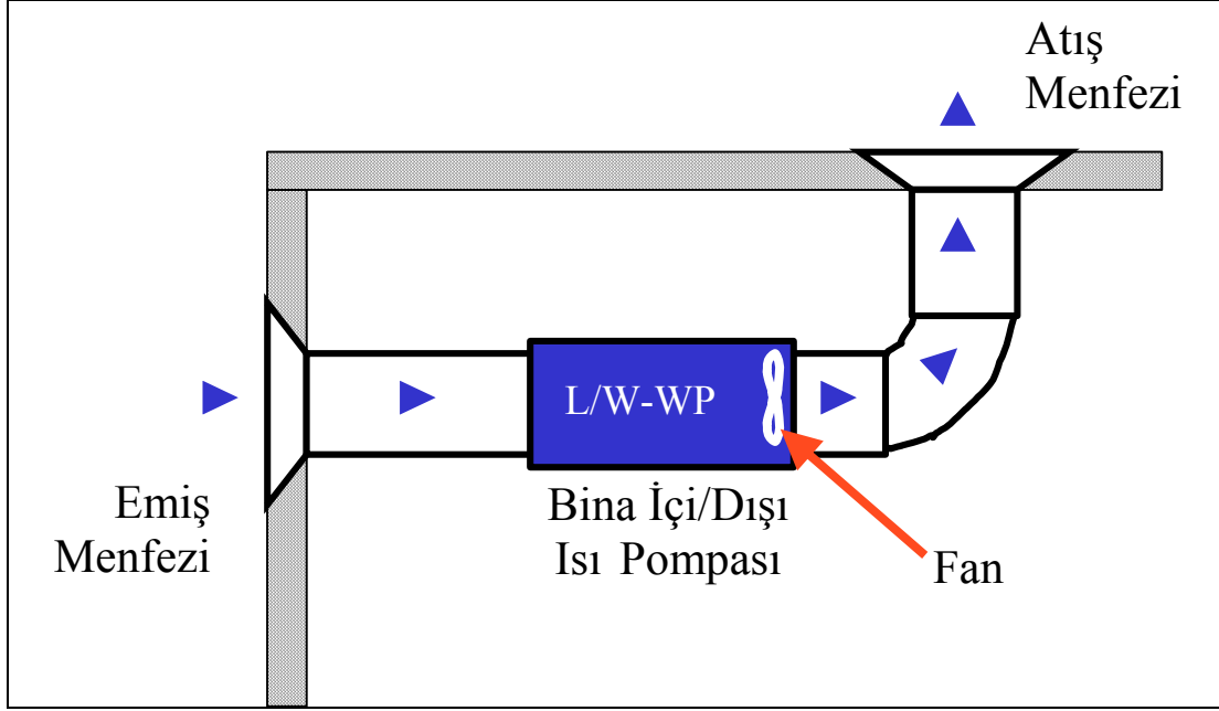
Şekil 6. Havadan suya ısı pompası bina içi tesisi şeması
