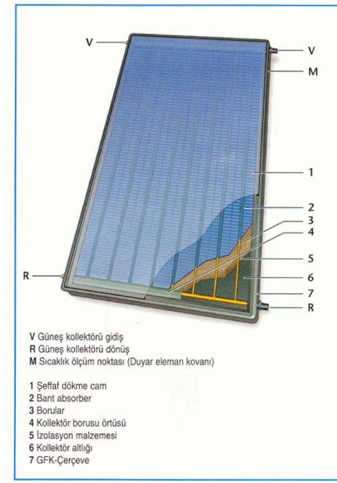
Şekil 12. Düzlemsel güneş kolektörleri
