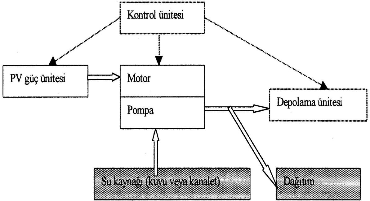
Şekil 1. PV Pompa Sistemi Bileşenlerinin Blok Diyagramı
