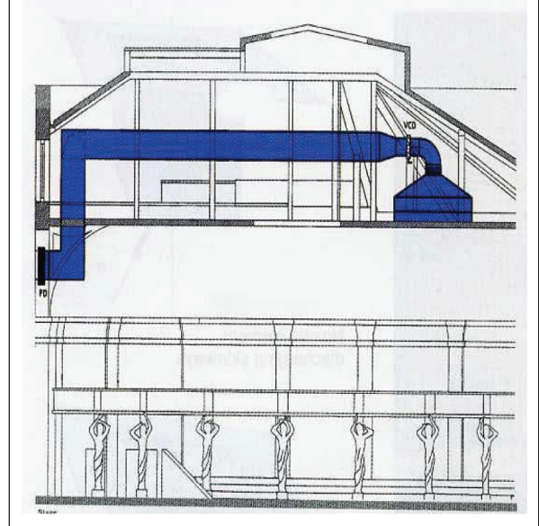
Şekil 12. Kesit
