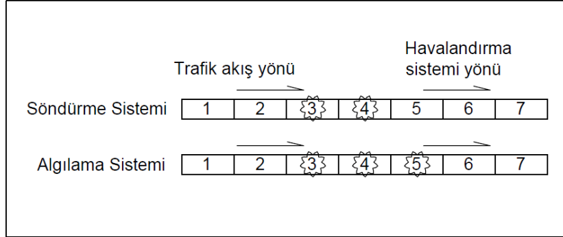
Şekil 1. Tek yön trafikli tünelde algılama ve söndürme sistemi: 3, 4 ve 5 zonlarından gelen algılama sinyaliyle sistem, 3 ve 4 zonlarında yangın çıktığına karar vererek bu zonlardaki söndürme sistemlerini çalıştırıyor.
