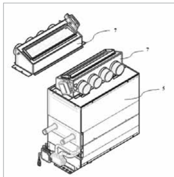
Şekil 4. Modüler Defroster Komponenti
