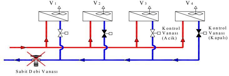
Şekil 20. Sabit Debi Vanasının Yanlış Kullanım Şekli
