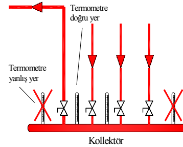
Şekil 2. Kollektör Termometre Yerleşimi
