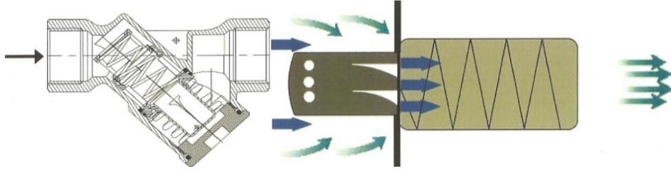
Şekil 15. Dinamik Kartuşlu Sabit Debi Vanası[3]
