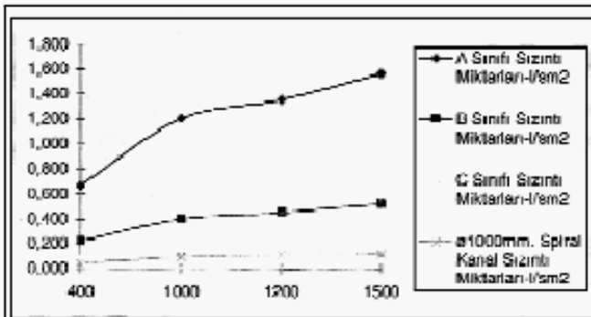
Şekil 7. Silindirik Kanal (Ø 1000mm) için Hava Sızıntı Miktarları.
