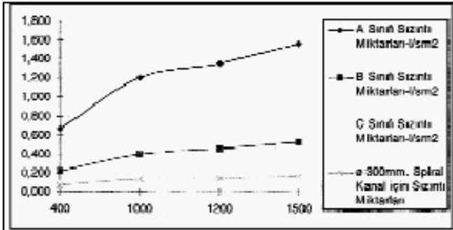
Şekil 6. Silindirik Kanal (Ø 300mm) için Hava Sızıntı Miktarları.
