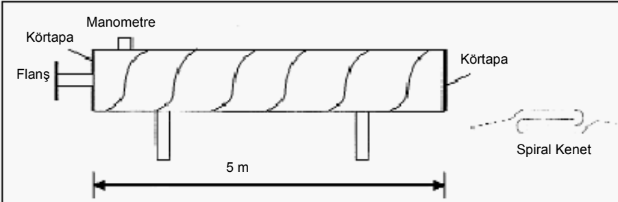
Şekil 2. Spiral Kanal Test Montajı ve Yivli Kenet Detayı [7].
