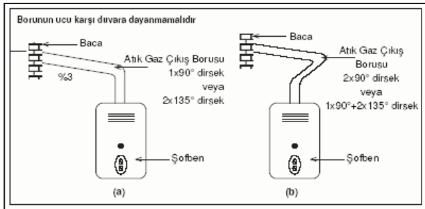
Şekil 4: Şofben baca bağlantı detayı
