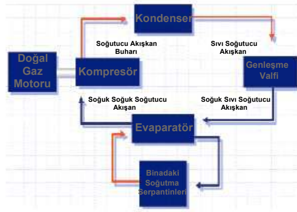
½ekil 6. Doğalgaz motor tahrikli Çiller şeması[2]
