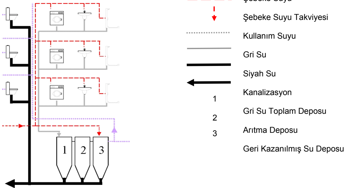
Şekil 2. Standart Gri Su Geri Kazanım Sisteminin Kurulum Şeması. (Kazanılan Su Kullanım Suyu Olarak Çamaşır Makinesinde ve Bahçe Sulamada da Kullanılabilir).
