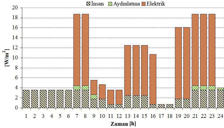
Şekil 5. İç Isı Kazançları [W/m 2 ] Günlük Profili
