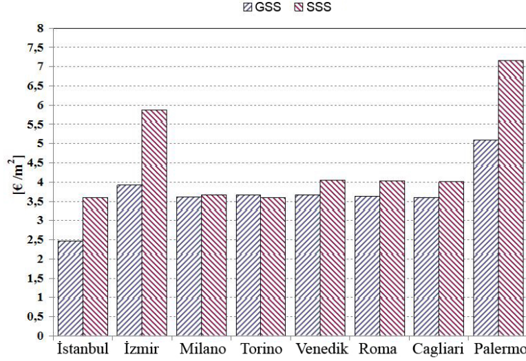
Şekil 9. Geleneksel Soğutma Sistemi ve Solar Soğutma Sisteminin Yıllık Sıcak Su Üretimi ve Yaz Dönemi Soğutma Maliyetlerinin 25 Yıllık Ortalamaları
