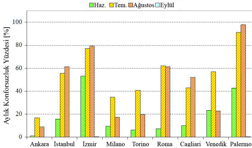
Şekil 6. Soğutma Sistemi Olmadığı Koşuldaki İç Hava Konforsuzluğunun Aylık Yüzdeleri
