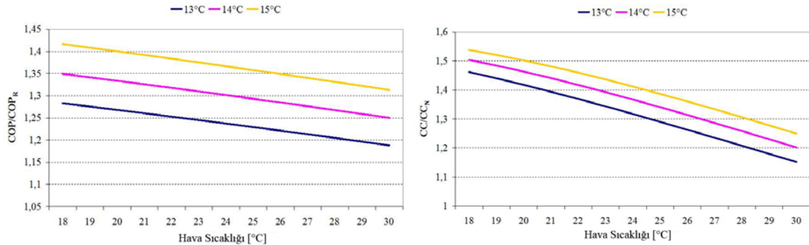
Şekil 3. (a) COP [-] ve Soğutma Kapasite [-]
