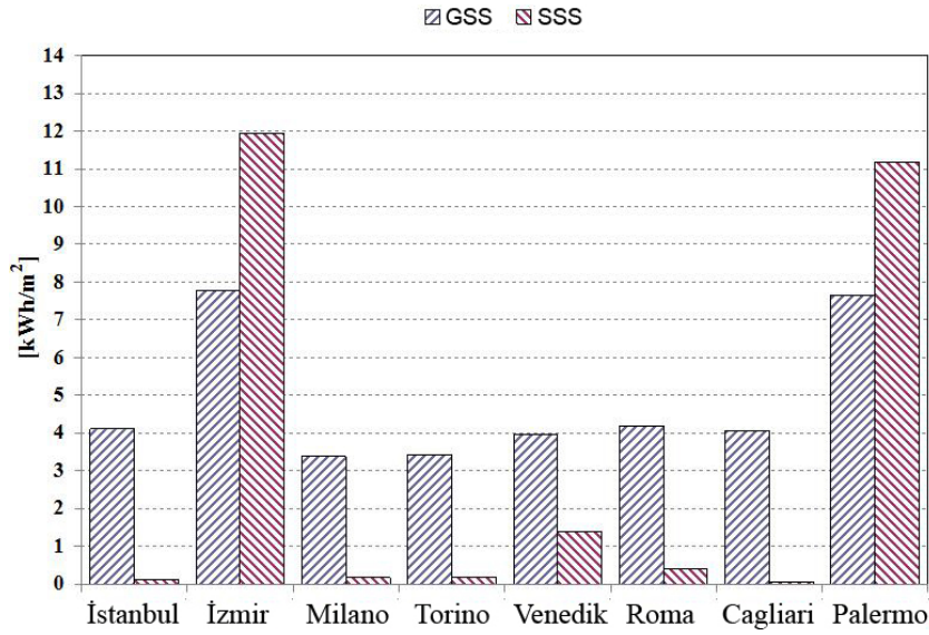
Şekil 7. Yıllık Sıcak Su Üretimi ve Yaz Soğutması: Geleneksel ve Güneş Destekli Sistemlerin Birincil Enerji Tüketimleri [kWh/m 2 ]
