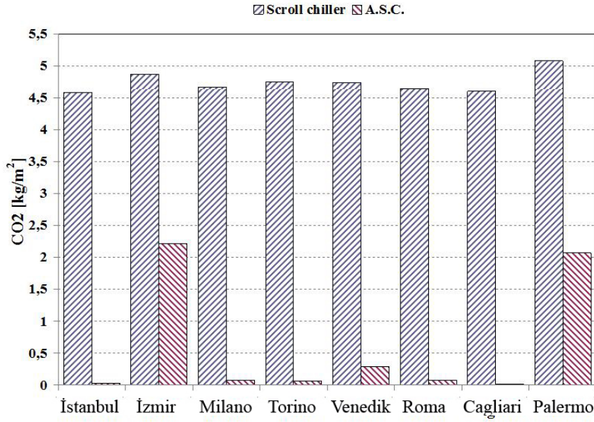
Şekil 8. Geleneksel ve Güneş Destekli Soğutma Sistemlerinin Yıllık Sıcak Su Üretimi ve Yaz Soğutması Süresince Oluşan Karbondioksit Emisyonları [ kg/m^2 ].
