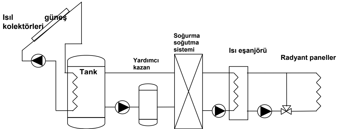
Şekil 1. Güneş Soğutma Santrali Şeması
