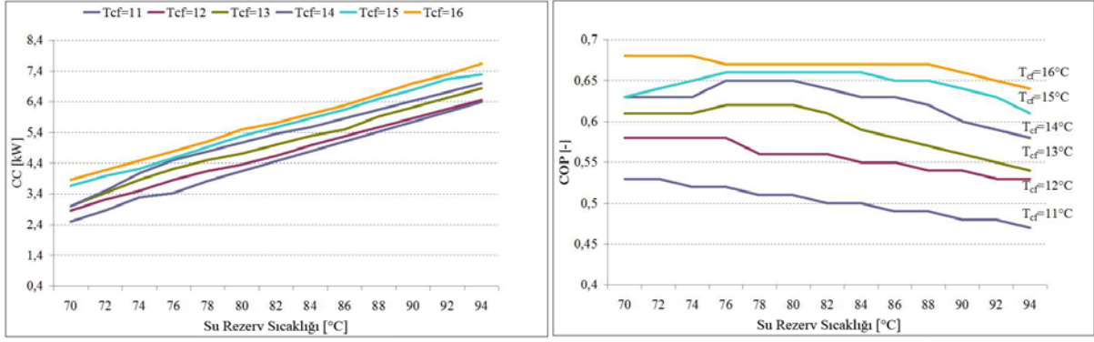
Şekil 2. (a) Soğutma Kapasitesi (kW)
