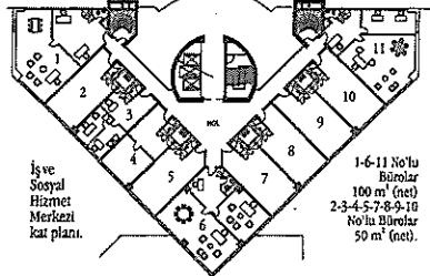
50 ve 100 m'lik bürolarda kullanıma örnek yerleşim planı.
