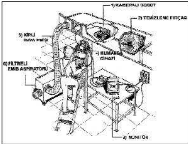
Şekil 1. Mekanik temizlik işlemi ekipmanları
