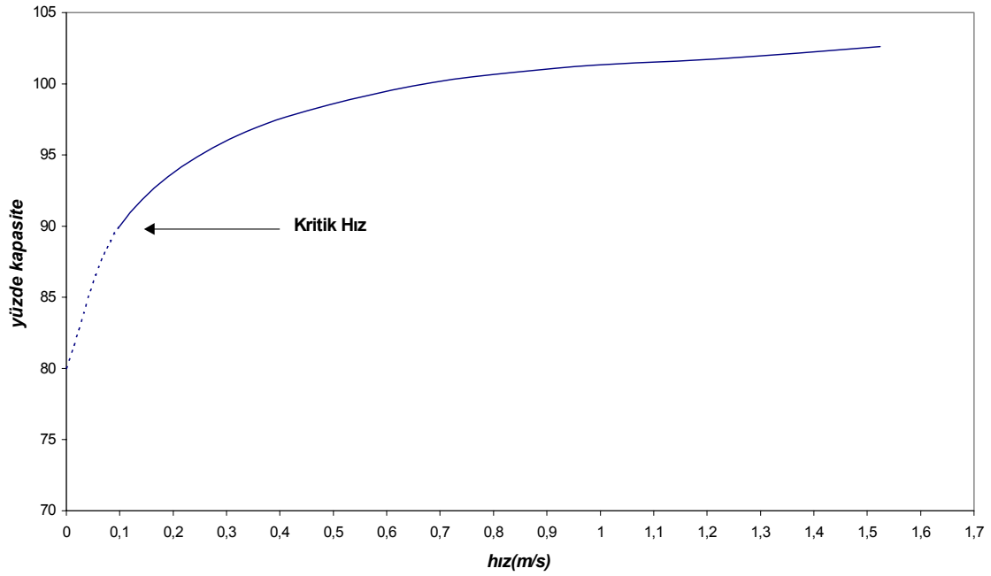
Şekil 1. Su ısıtma sistemlerinde düşük su hızlarının ısı transferine olan etkisi
