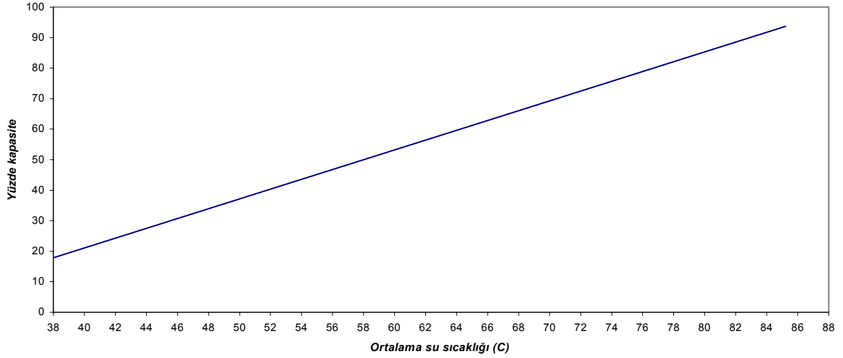
Şekil 2. Düşük su sıcaklıkları için ortalama kapasite
