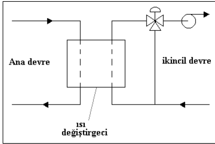
Şekil 5. Jeotermal akışkanı bina ısıtma sisteminden ayırmak için kullanılan ısı değiştirgeci sistemi
