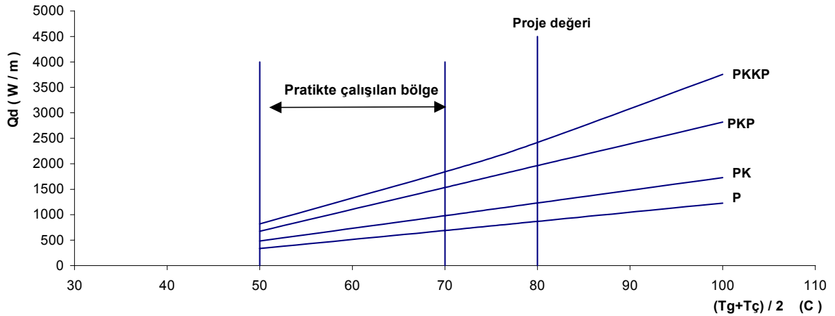
Şekil 3. 600 mm. Yüksekliğindeki panel radyatör tiplerinin ısı kapasite eğrileri
