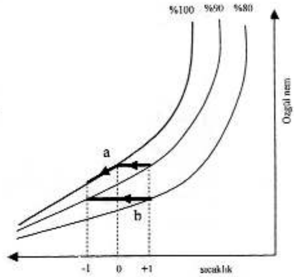
Şekil 4. Soğutucu üniteye Azkarlama olması veya yoğuşma olmaması
