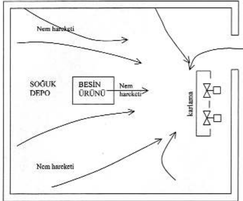
Şekil 2. Soğutucu ünite de karlama olayına neden olan nem hareketi
