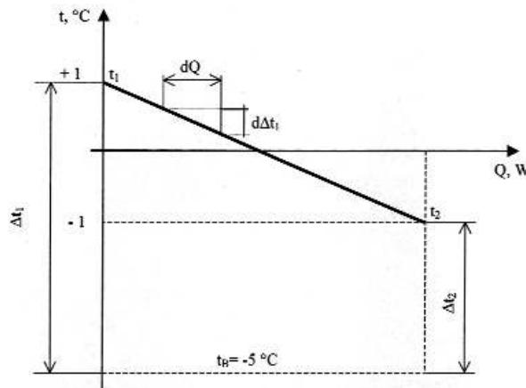
Şekil 7. Soğutucu üniteye logaritmik ortalamaya esas sıcaklık değişimleri
