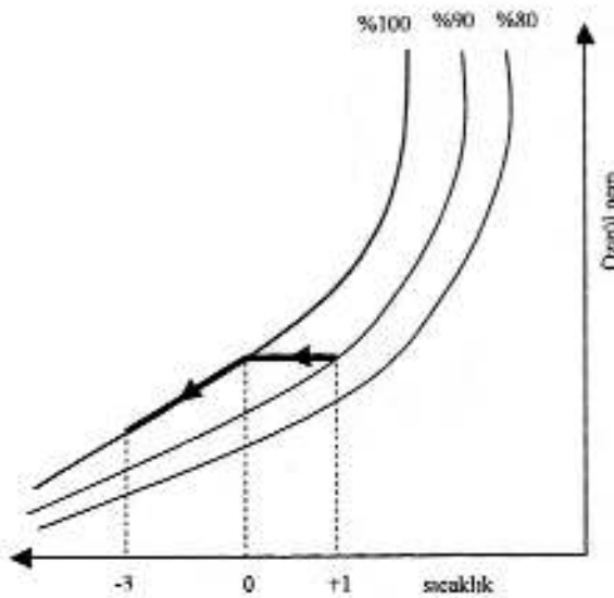
Şekil 3. Soğutucu üniteye aşırı karlama olması
