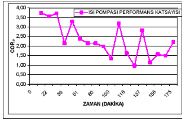
Şekil 4.2. Parçalı Bulutlu Hava İçin COP IP Değişimi
