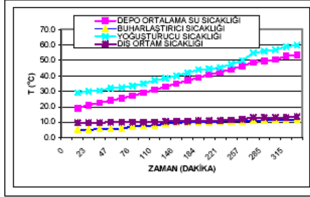
Şekil 4.7. Sağanak Yağmurlu Hava İçin Sıcaklık Değerleri Değişimi
