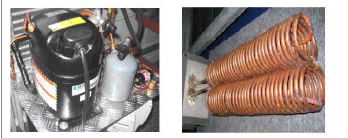
Şekil 3.3. Kompresör, Sıvı Deposu, Filtre Kurutucu ve Gözetleme Camı, Helisel Kıvrılmış Yoğuşturucu Kompresörden çıkan basıncı ve sıcaklığı yüksek çevrim akışkanı yoğuşturucuda ısıyı suya vererek yoğuşturucu çıkışında sıvı deposunda (1 litre) toplanır. Sıvı deposu çıkışı ¼ boruyla kaynaklı bağlantılı filtre (0,035litre), kurutucu ve nem gösterme kapasiteli gözetleme camı mevcuttur.
