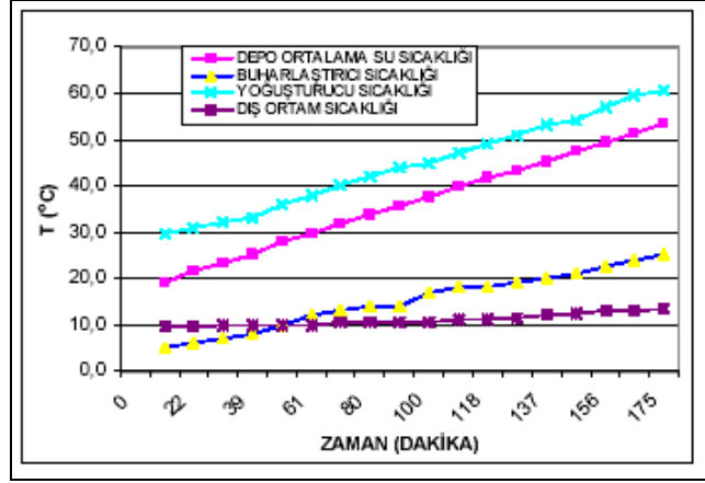
Şekil 4.1. Parçalı Bulutlu Hava İçin Sıcaklık Değerleri Değişimi
