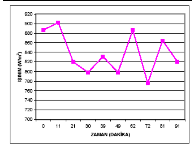
Şekil 4.6. Açık Güneşli Hava İçin Işınım Değerleri Değişimi
