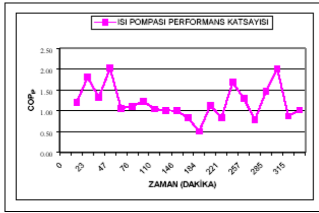
Şekil 4.8. Sağanak Yağmurlu Hava İçin COP IP Değişimi
