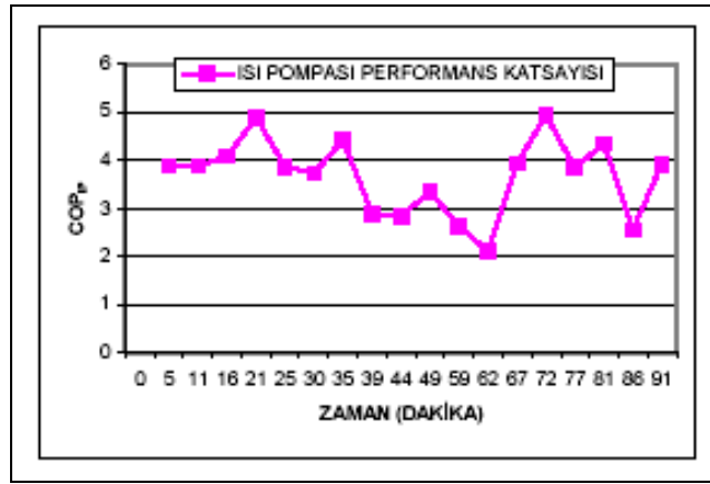
Şekil 4.5. Açık Güneşli Hava İçin COP IP Değişimi
