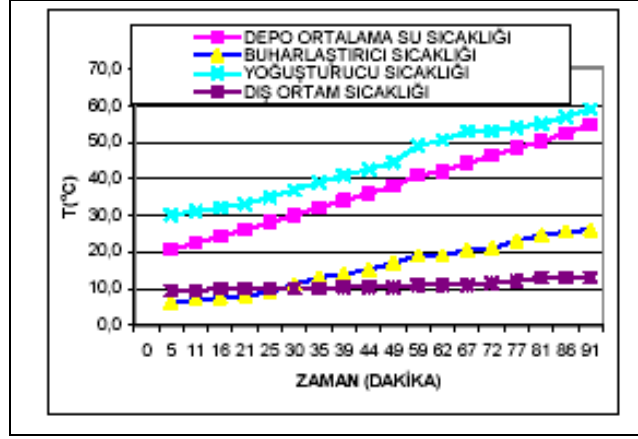
Şekil 4.4. Açık Güneşli Hava İçin Sıcaklık Değerleri Değişimi
