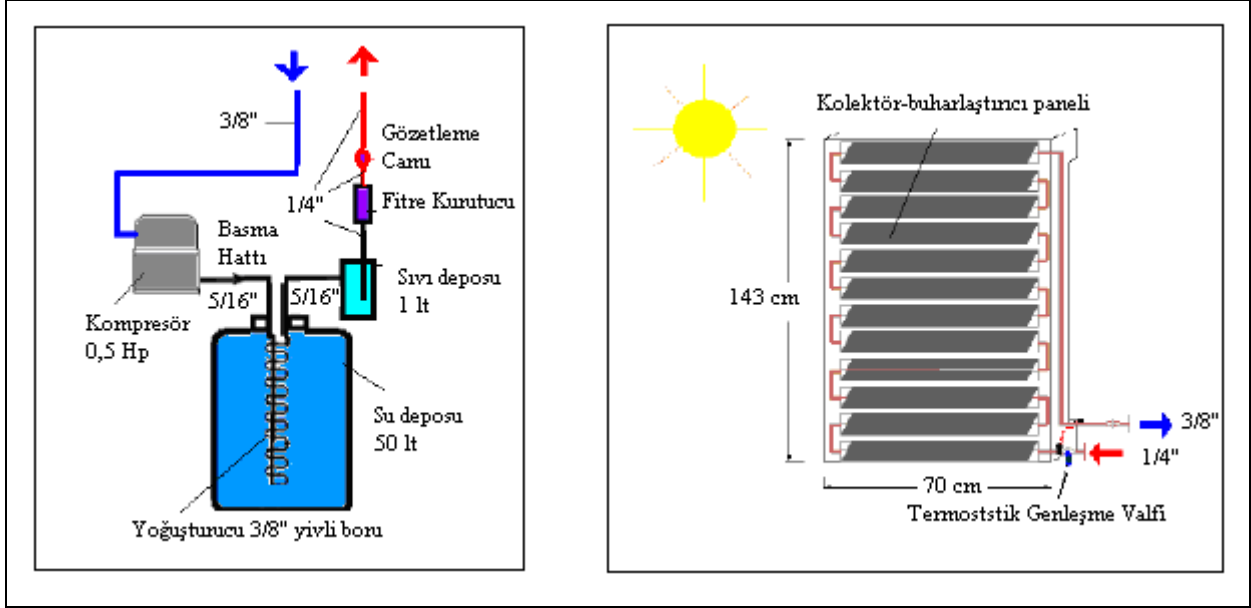
Şekil 3.1. Isı Pompası İç ve Dış Ünite Temel Şeması
