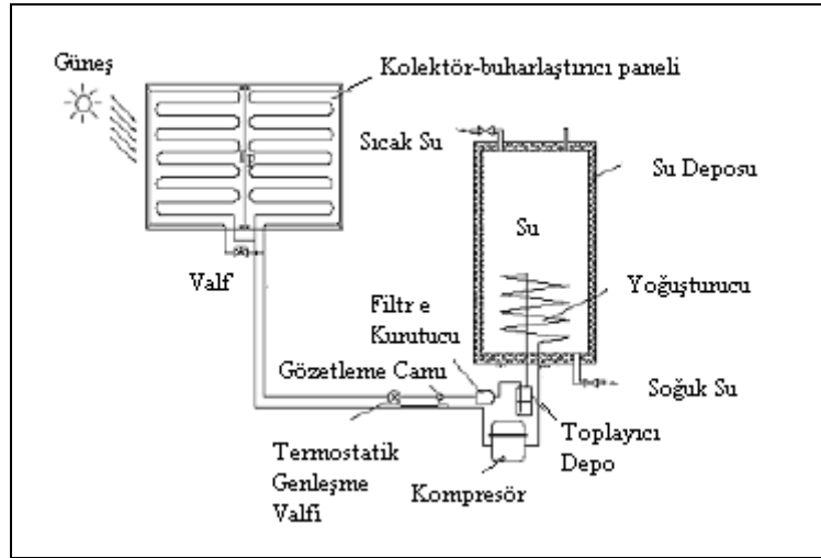
Şekil 2.1. Direkt Genişmeli Isı Pompalı Su Isıtıcısı Temel Bileşenleri
