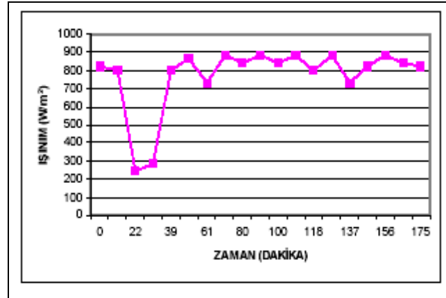
Şekil 4.3. Parçalı Bulutlu Hava İçin Işınım Değerleri Değişimi
