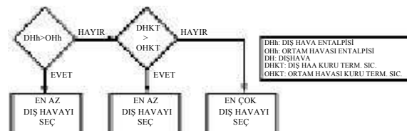
Şekil 10. Entalpi seçim diyagramı [10]
