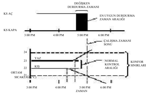
Şekil 6. En uygun durdurma [10]
