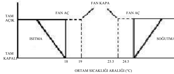
Şekil 9. Sıfır enerji bandında fan kontrolü [11]
