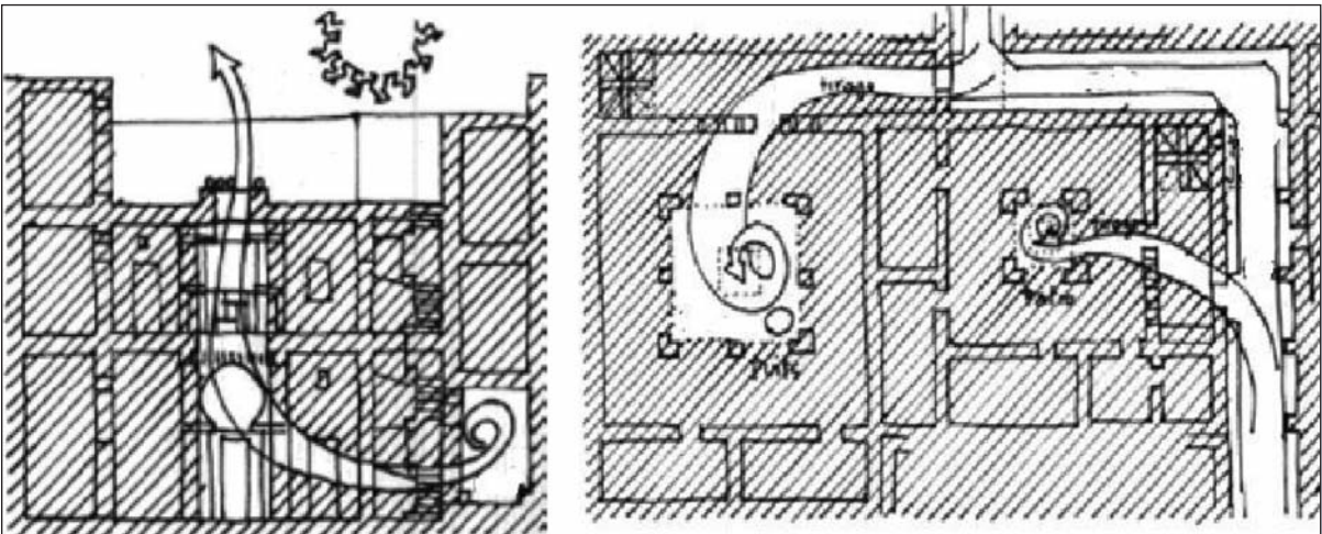
Şekil 8. Kasbash Konutunda Konveksiyon Yoluyla Havalandırmaı Gösteren Plan ve Kesit [17]
