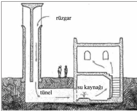
Şekil 9. Buharlaşma Etkili Rüzgâr Kulesi Tasarımı [17].
